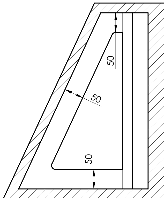
PRZEKRÓJ B-B
