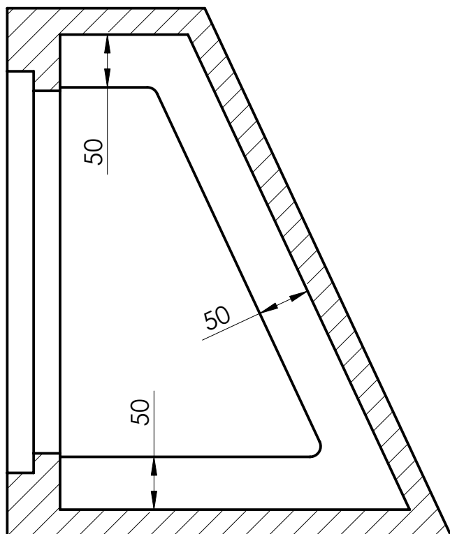
PRZEKRÓJ A-A
