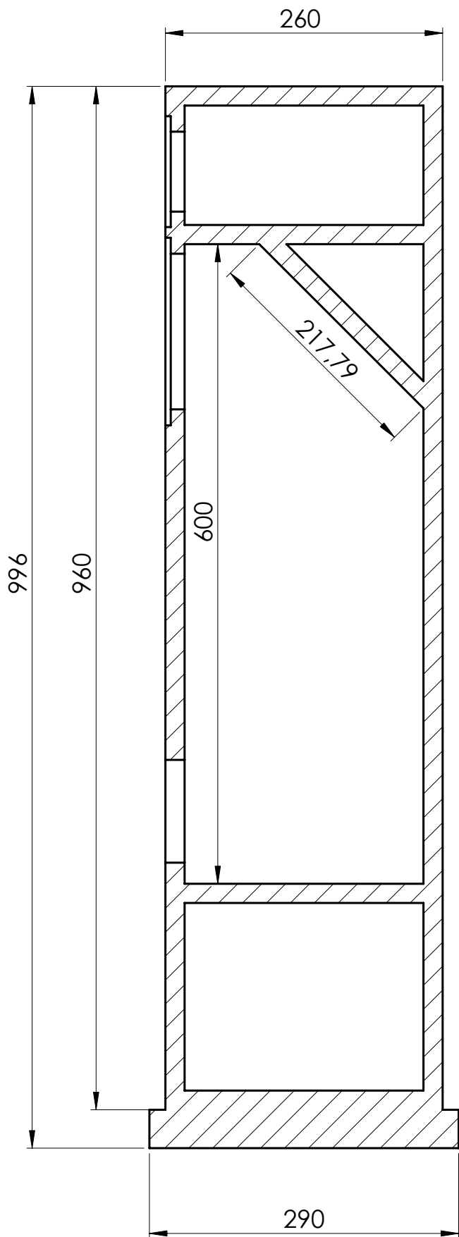
PRZEKRÓJ A-A SKALA 1 : 5
